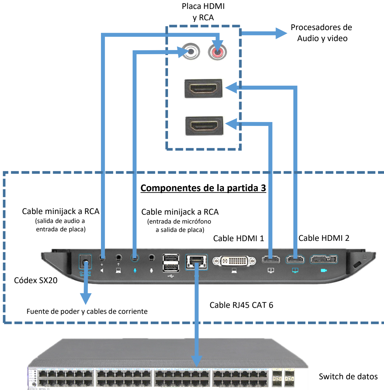
Diagrama de ubicación física y conexión del códec solicitado en el Anexo Técnico A, partida 3.
