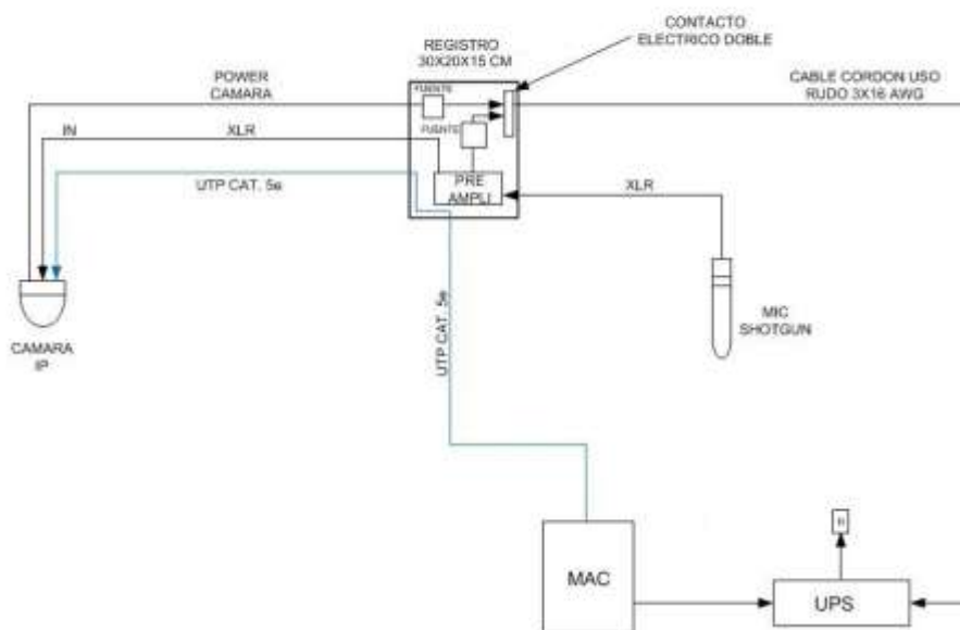
DIAGRAMA DE CONEXIÓN SALAS
