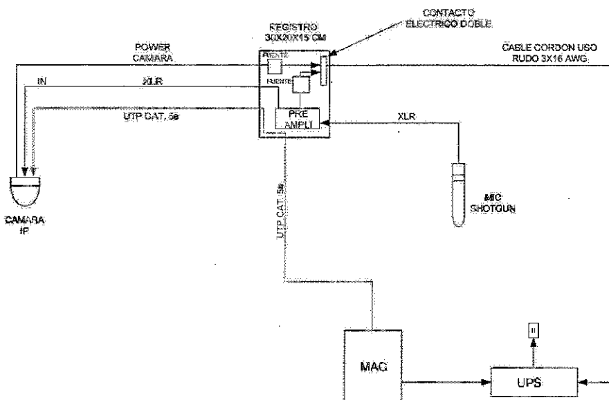
DIAGRAMA DE CONEXIÓN SALAS
