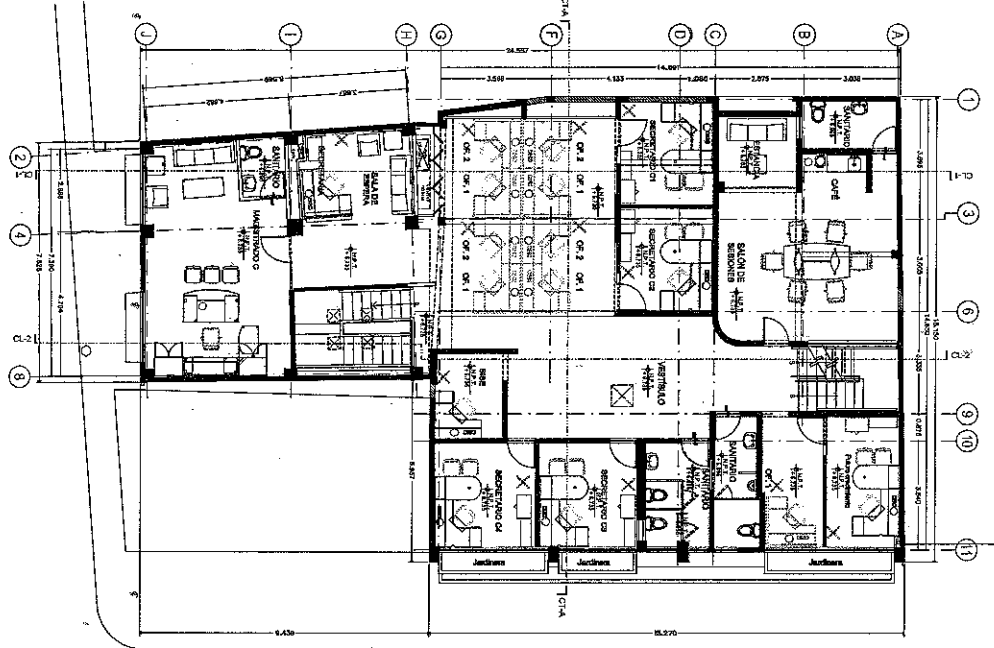
PLANTA 2o NIVEL
